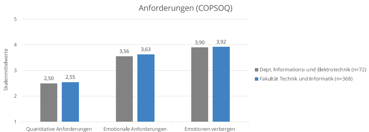
Abbildung 11: Verteilung der Anforderungen durch das Studium für das Department Informations- und Elektrotechnik und die Fakultät TI
